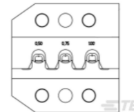
TE Teilnr.: 6-1579016-8 ERGO CRIMP DIE SET, INCL. LOCATOR, SKF 1.5
